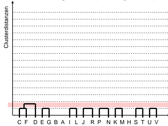
Dendrogram (Average Link)
