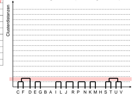
Dendrogram (Average Link)
