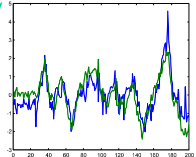
Offset Translation + Amplituden Skalierung + Lineare Trend Beseitigung
