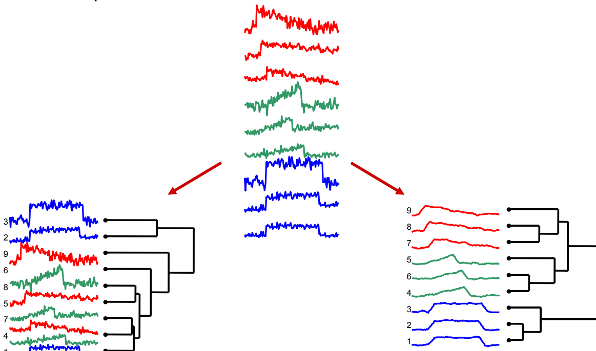
Hierarchisches Clustering mit Euklidischer Distanz nach Bereinigung von Rauschen, Beseitigung linearer Trends, Amplituden Skalierung und Offset Translation
