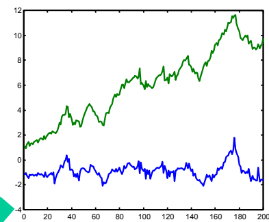
Offset Translation + Amplituden Skalierung
