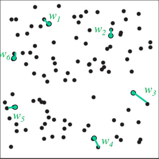
Zufallsauswahl aus Datensatz (m Punkte) m \ll n
