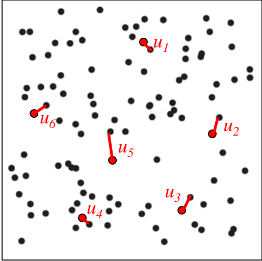
m gleichverteilte Punkte
