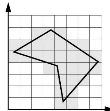
Rastermodell:
