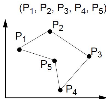
Vektormodell:
