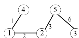
ein minimaler Spannbaum Gesamtkosten = 12
